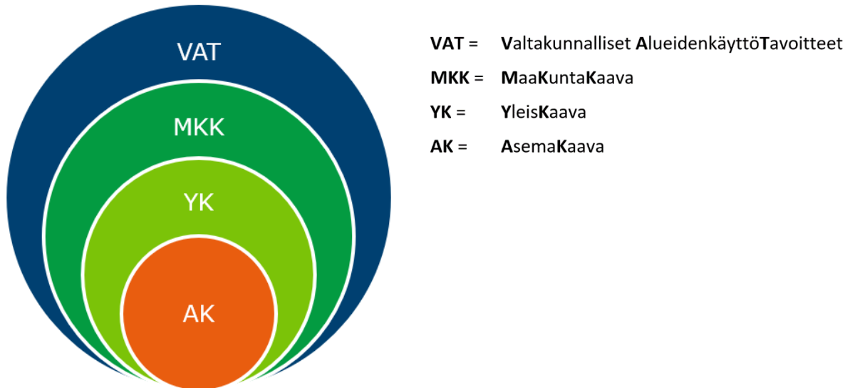
Kuva 9: Kaavahierarkia
